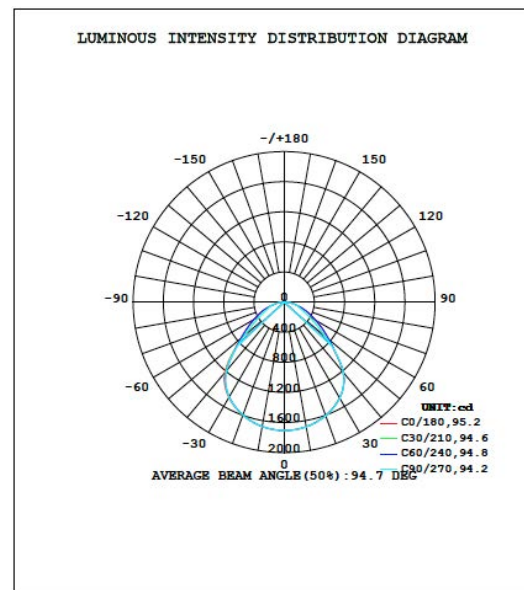
Lichtverteilung
