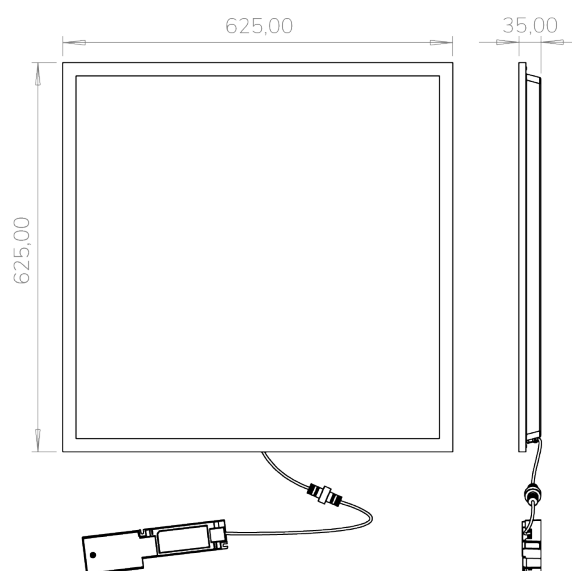
Maßzeichnung
