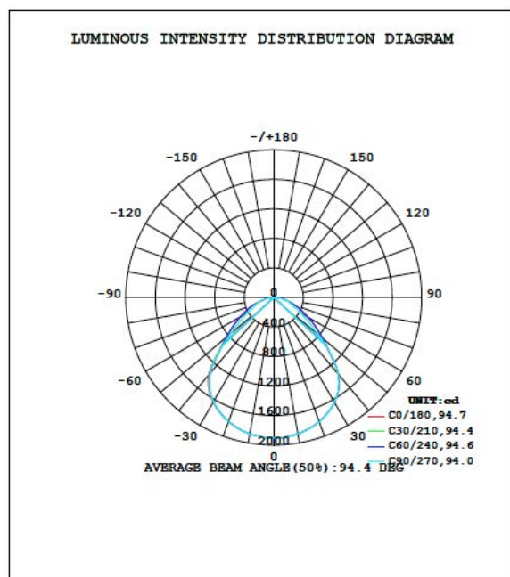
Lichtverteilung
