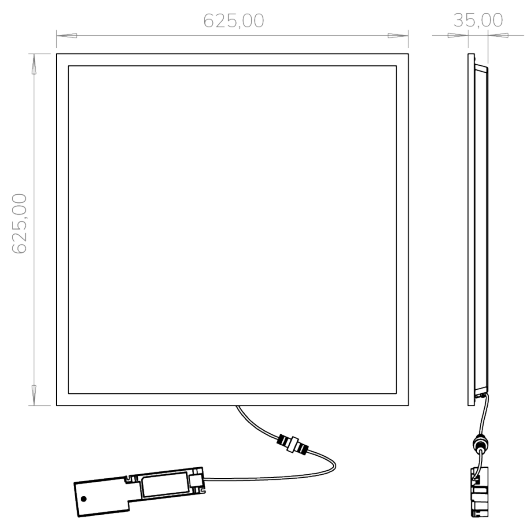
Maßzeichnung
