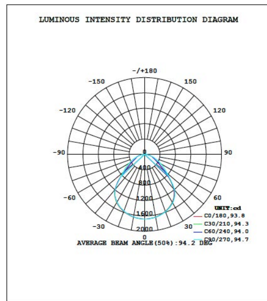
Lichtverteilung
