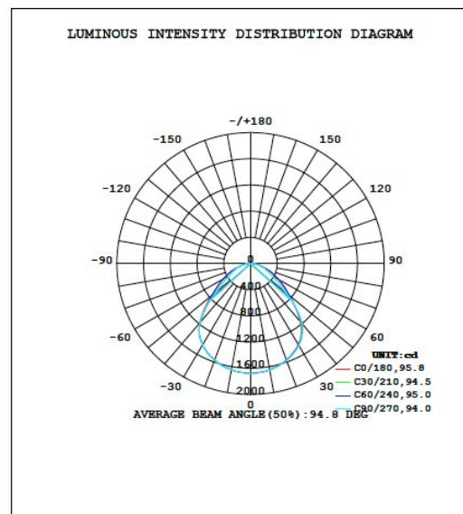
Lichtverteilung
