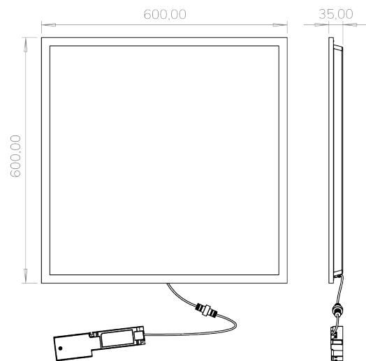
Maßzeichnung
