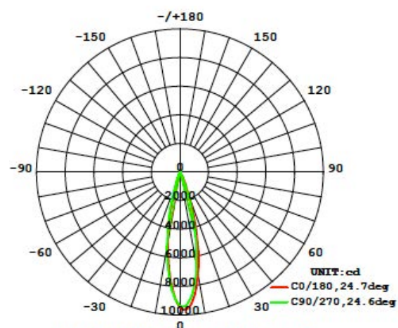
Lichtverteilung
