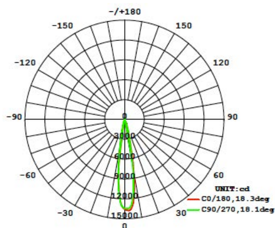
Lichtverteilung
