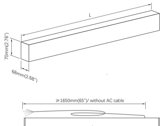
Maßzeichnung
