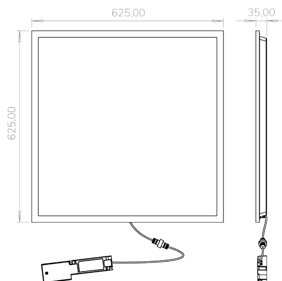
Maßzeichnung
