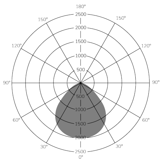
Lichtverteilung
