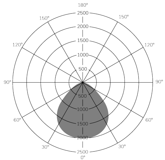
Lichtverteilung
